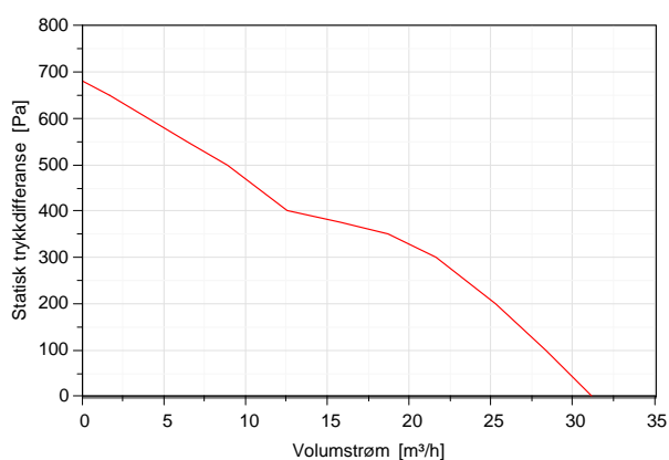
Figur 23. Viftenes karakteristikkt. Driftsområdet vil være i nedre høyre område der hvor dP_{stat} < \sim 300 Pa.
