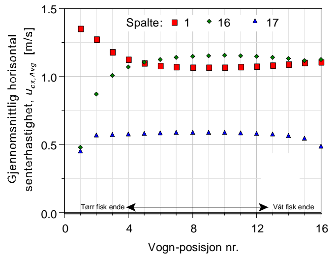
Figur 8. Gjennomsnittlig hastighet for vogner. Senterhastighet midt mellom brett for spalte 1 (mellom nederste og nest nederste brett) og spalte 16; For spalte 17: Over øverste brett, d.v.s. mellom øverste brett og vogntak er hastigheten ”målt” i samme høyde over fisk som for de øvrige brettene. Luftinnløp er i tørr ende, utløp i våt ende.
