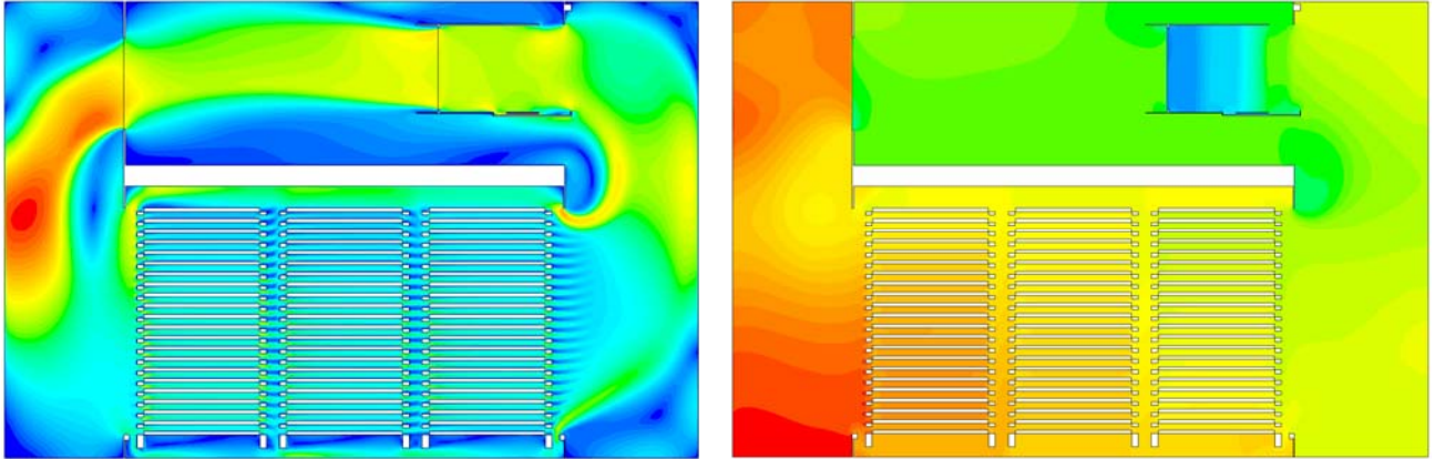
Figur 24. Resultat av Fluent-simulering av viskøs, isoterm strømming. Hastighetsfelt til venstre ( 0 < u < 8,5 m/s) og statisk trykkfelt til høyre ( -220 < P < 5 Pa).
