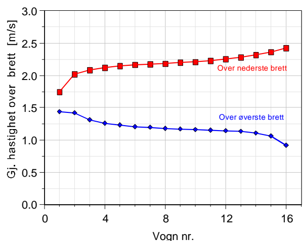
Figur 18. Beregnet forandring av lufthastighet langs tunnelen i spalter over henholdsvis nederste og øverste brett. Dette er middelverdier for vognene målt i en høyde over fisken som tilsvarer senterposisjon mellom to fiskebrett.
