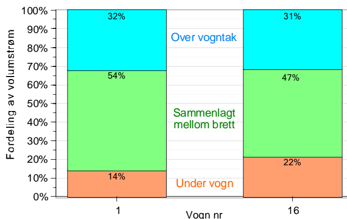
Figur 11. Beregnet fordeling av luftstrømmen under, gjennom og over første og siste vogn i rekken. Beregnet fra hastighetsprofil midt gjennom hver vogn.
